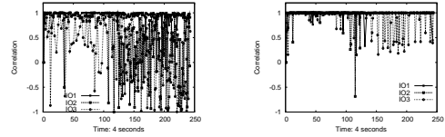
(c) corr(req, interrupt) (d) corr(iosize, svctm)
