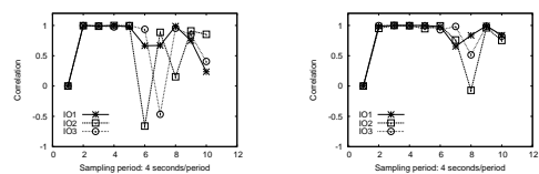
(c) corr(req, interrupt) (d) corr(iosize, svctm)
